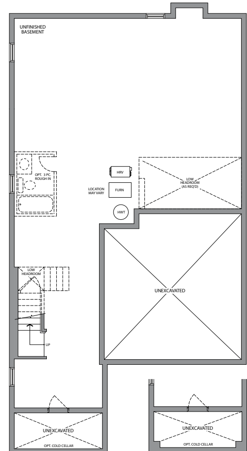
BASEMENT STYLE 'B'
