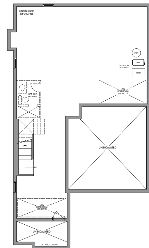
BASEMENT STYLE 'B'
