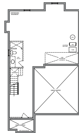
BASEMENT STYLE 'A' & 'B'
